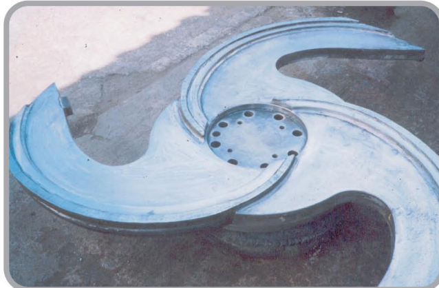
เชื่อมใบพัดผสมเยื่อ พอกผิวแข็งพร้อมทำบาลานซ์
